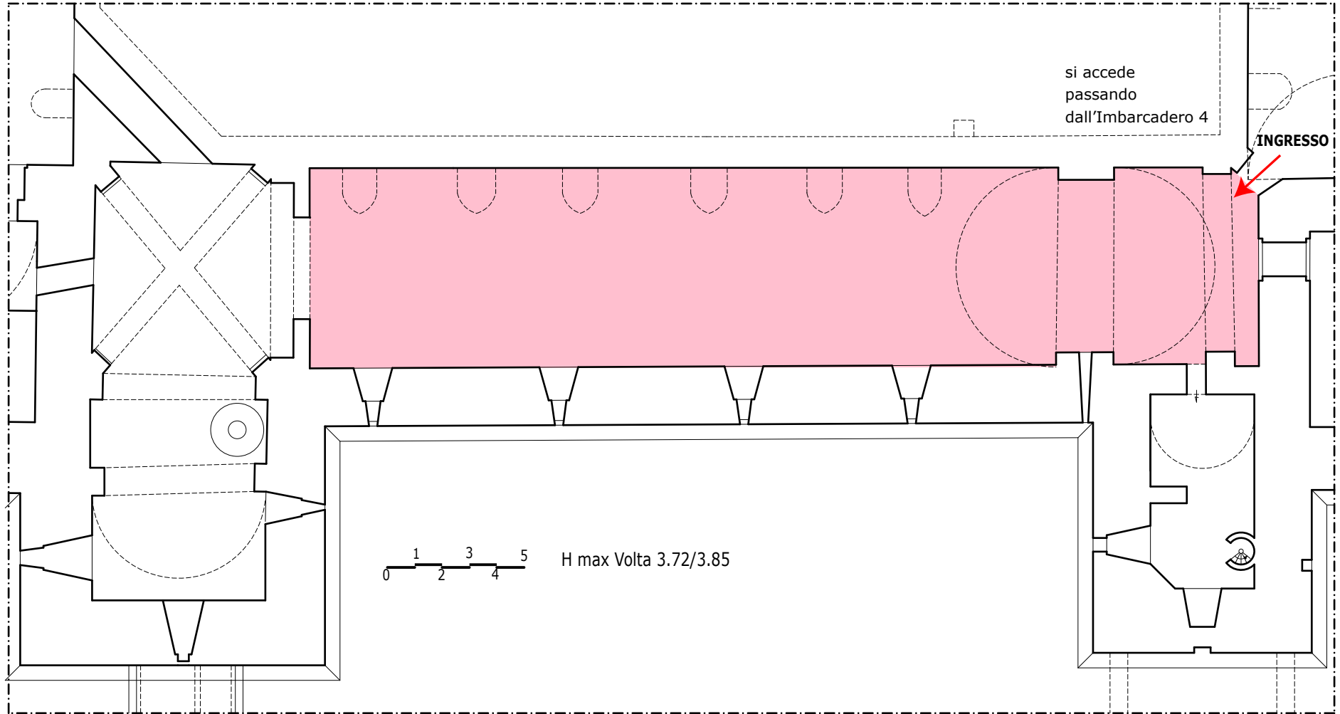
PIANTA
